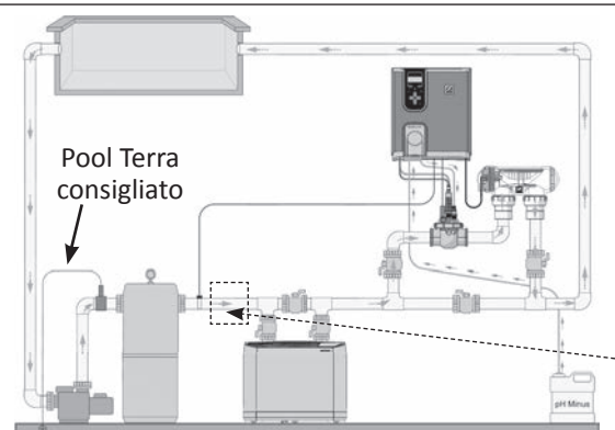
Installazione con un sistema di riscaldamento
